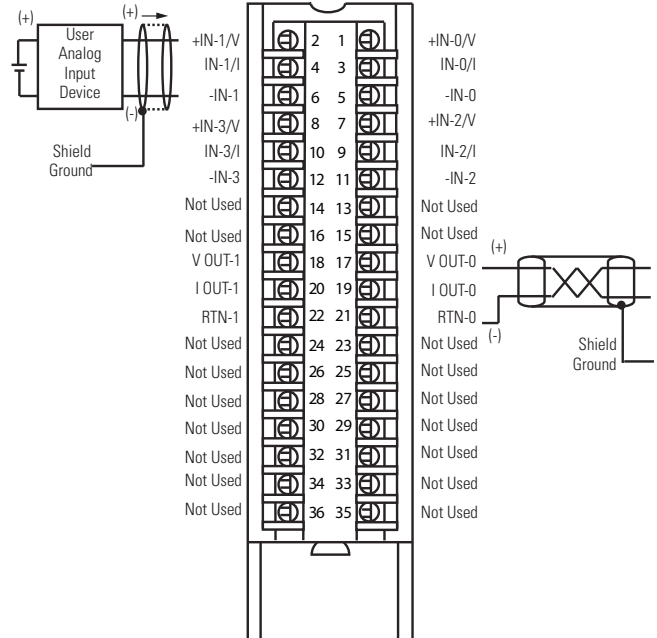
1756-IF4FXOF2F Voltage
